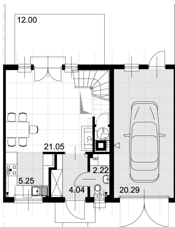
RZUT PARTERU
