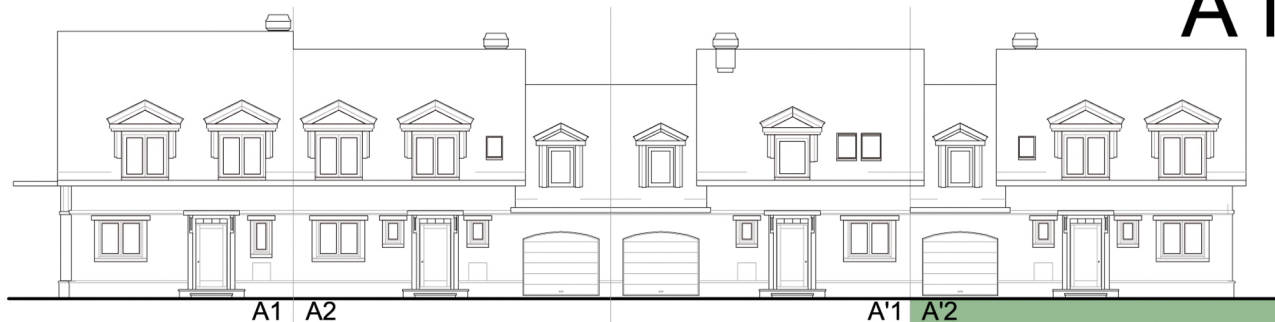
ELEWACJA FRONTOWA / WSCHODNIA
