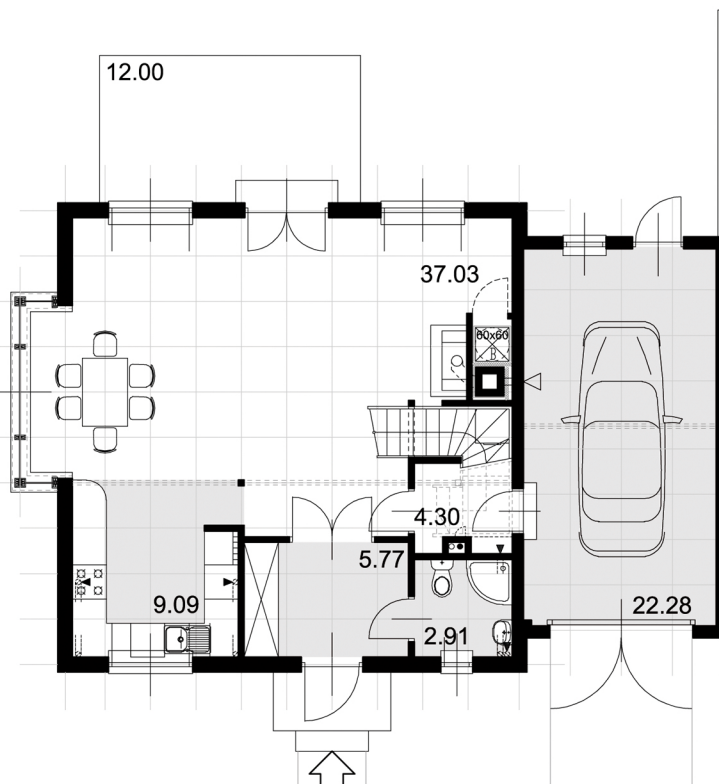
RZUT PARTERU
