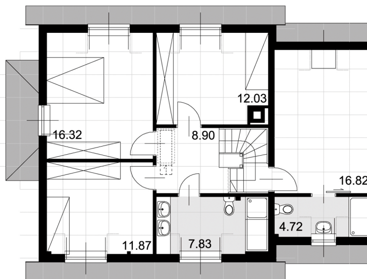
RZUT PIĘTRA
