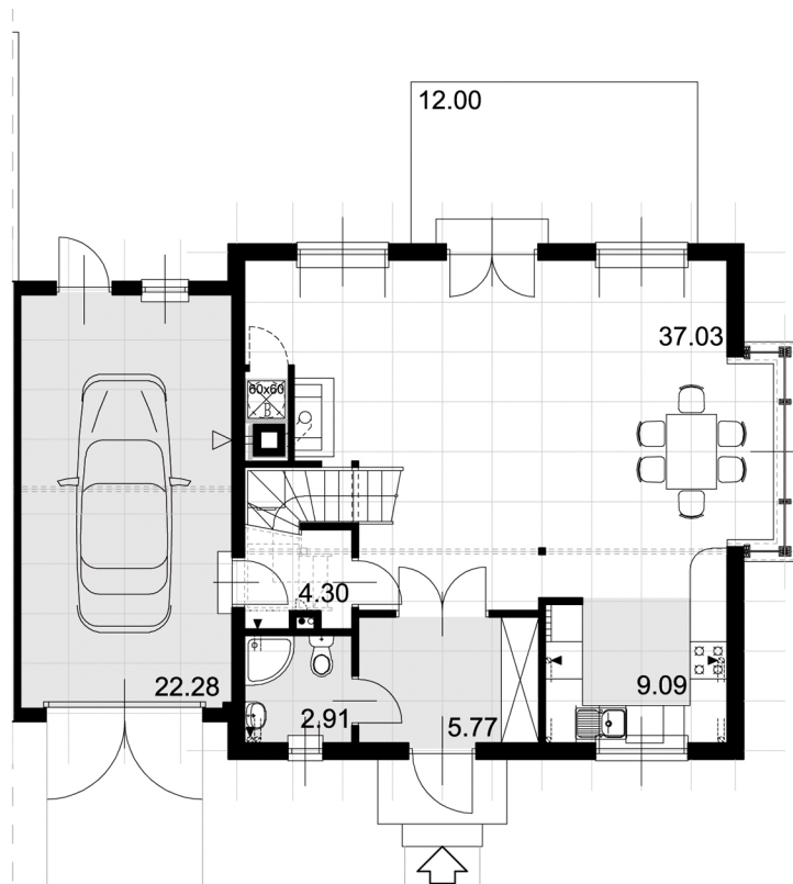
RZUT PARTERU
