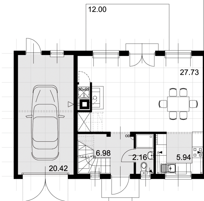
RZUT PARTERU
