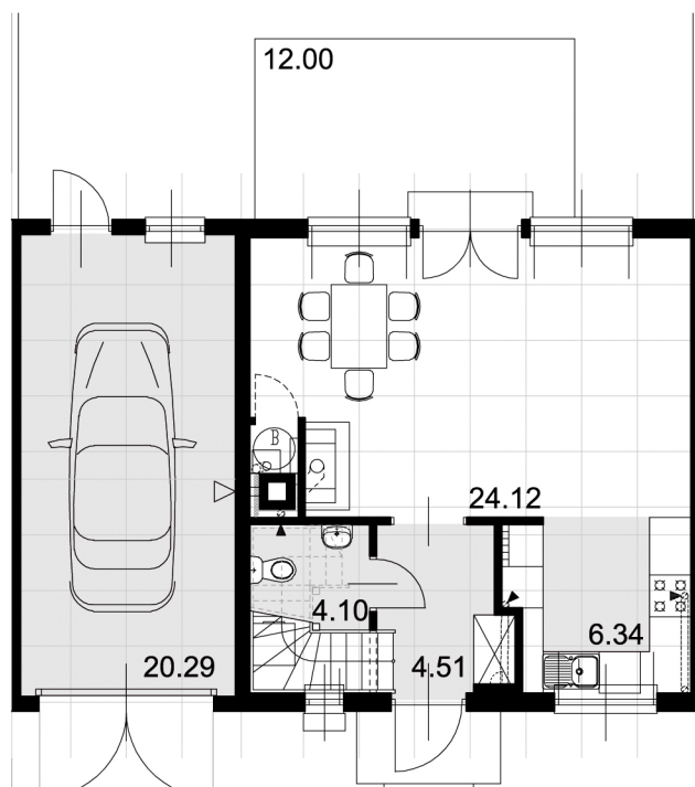
RZUT PARTERU
