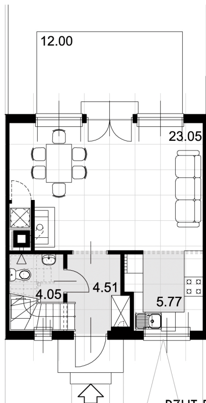
RZUT PARTERU
