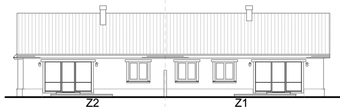
ELEVACJA OGRODOWA - POŁUDNIOWO ZACHODNIA
