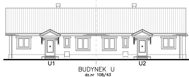
ELEWACJA FRONTOWA I OGRODOWA
