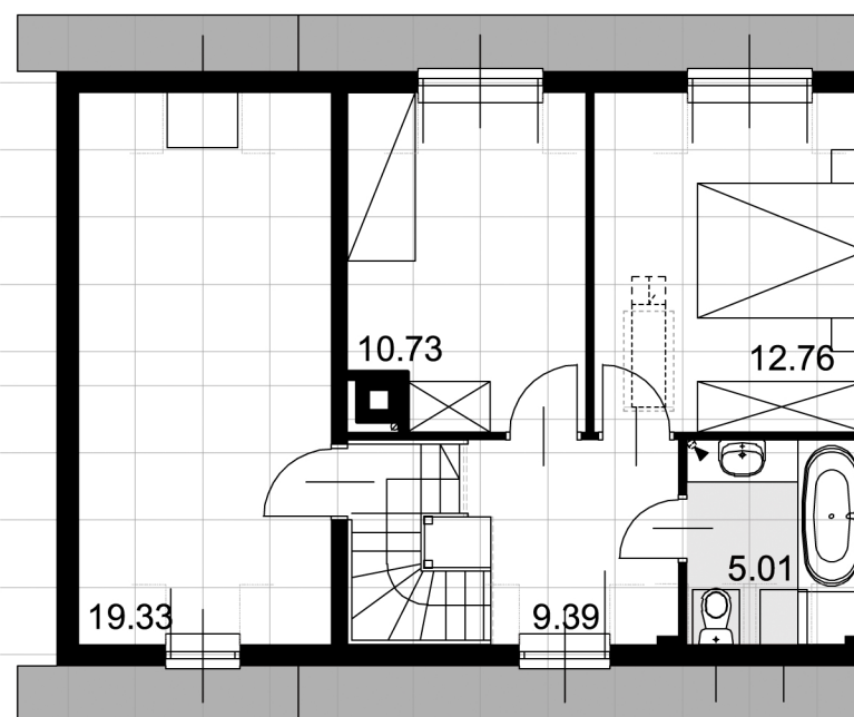
RZUT PIĘTRA 58,97 m² (50,81)
