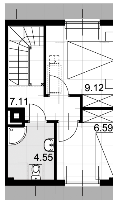
RZUT PIĘTRA 29,06 m 2 (26,96)
