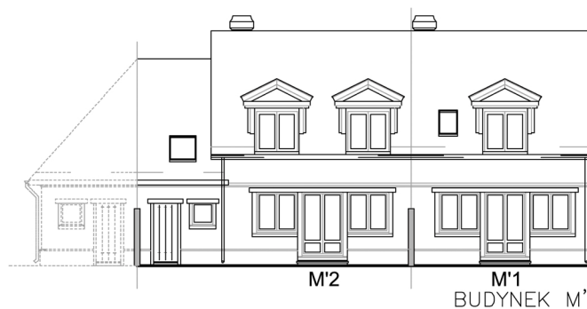
ELEWACJA FRONTOWA I OGRODOWA
