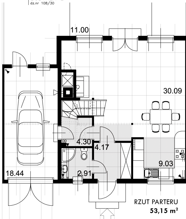
BUDYNEK L dz.nr 108/30
