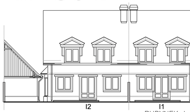
BUDYNEK I ELEWACJA FRONTOWA I OGRODOWA
